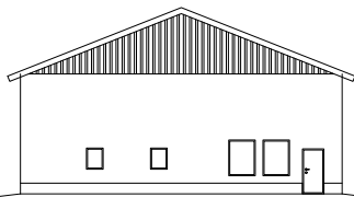
JULKISIVU ITÄN 1:100
